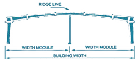
Multi Span "1" (MS-1)
