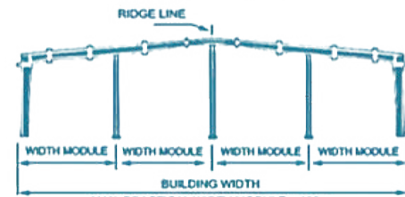
Multi Span "3" (MS-3)
